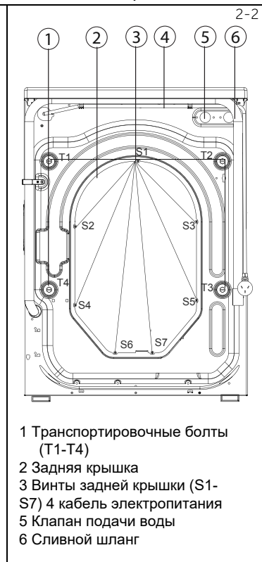
Задняя часть (рис. 2-2):
